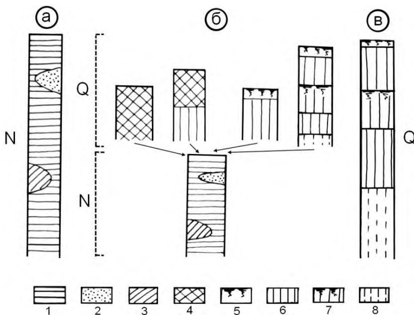
Рис. 2. Геологічні розрізи схилів балки між вул. Кармелюка і Старокостянтинівським шосе, м. Хмельницький (схематична узагальнена інформація за даними вишукувань «Хмельницький-будрозвідування» та «Житомирбудрозвідування» 1988–2017 рр.) [4]: а – неогенові відклади, б – четвертинні та неогенові відклади, в – четвертинні відклади; 1–3 морські відклади (1 – глини, 2 – піски, 3 – суглинки); 4 – насипні відклади, 5 – сучасний ґрунт, 6–8 – лесово-ґрунтова серія (6 – суглинки, 7 – викопний ґрунт, 8 – супіски).
