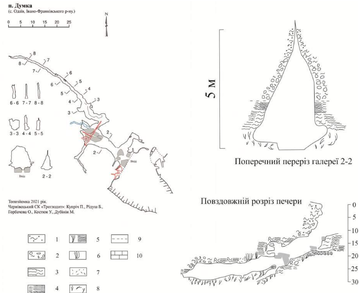
Рис. 1. Топографічний план печери Думка, поперечний переріз галереї (2-2) та поперечна проекція печери
