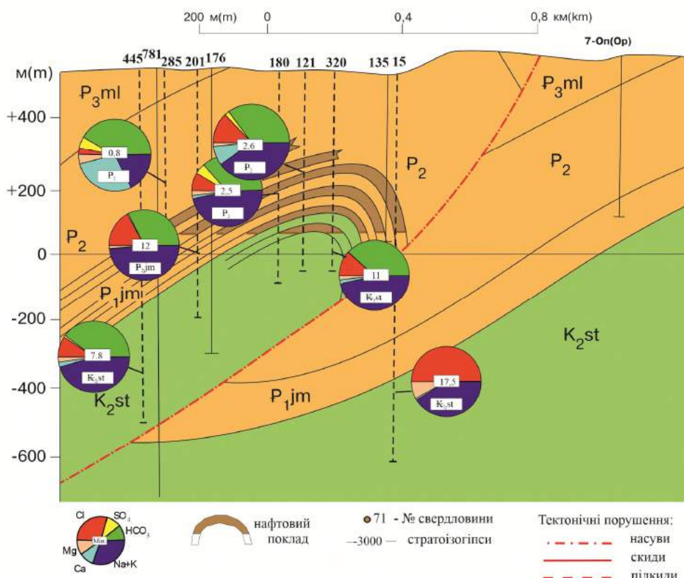
Рис. 2. Гідрогеохімічний профіль Східницького нафтового родовища (геологічна основа за Н. М. Хомяю, Л. П. Дідик [1])
