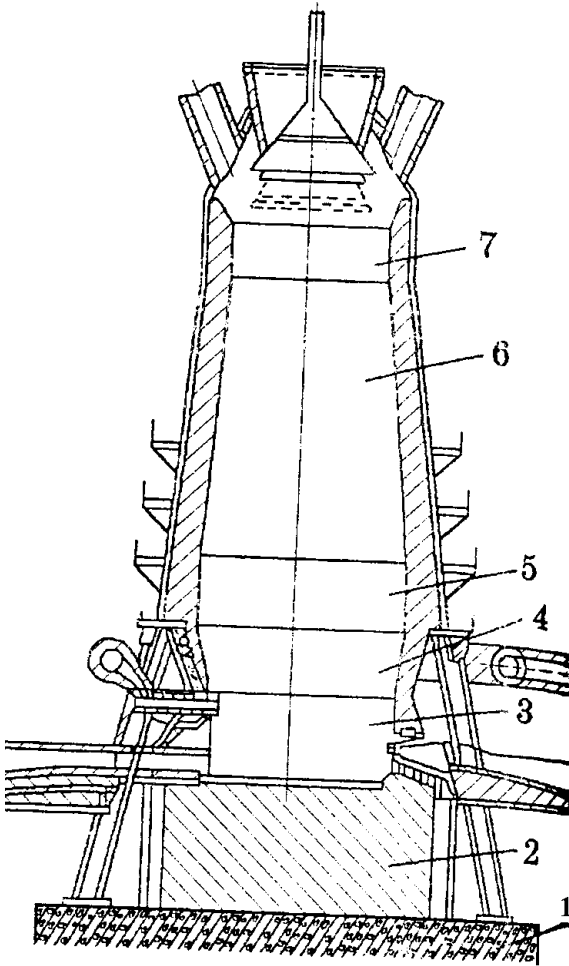
1 – фундамент; 2 – лешадь; 3 – горно; 4 – заплічники; 5 – розпар; 6 – шахта; 7 – колошник.
