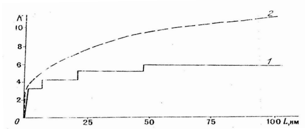
Рис. 3. Зміна порядку (K) річкової системи басейну р.Ріка за моделями Хортон - Штраллера (1) і Шайдеггера (2).
