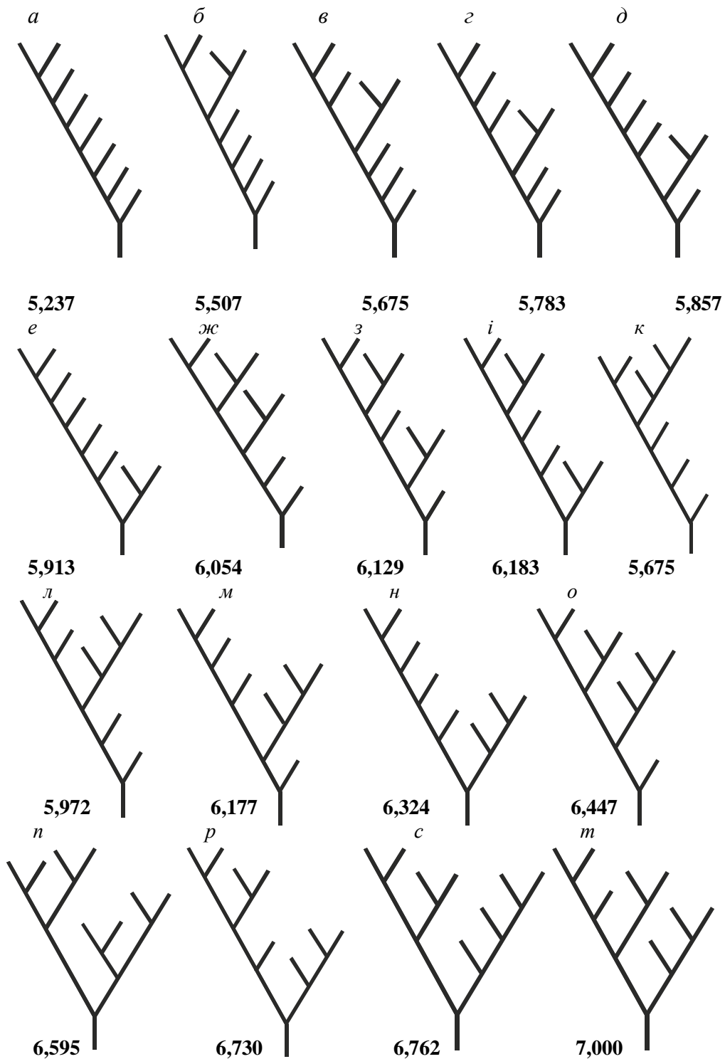
Рис. 6. Приклади різних за топологією річкових структур при S_d = 8 Цифрами вказані значення структурної ентропії H
