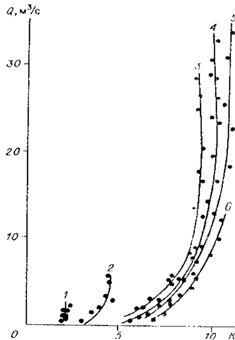
Рис. 5. Зв'язок середніх багаторічних витрат води ( Q ) із порядком ріки ( K ) для різних значень гідроморфологічного коефіцієнту (ГМК) Значення ГМК ( \text{км} \times \text{сек} / \text{м}^3 ): 1) 0 – 10; 2) 11 – 20; 3) 21 – 30; 4) 31 – 50; 5) 51 – 60; 6) >60
