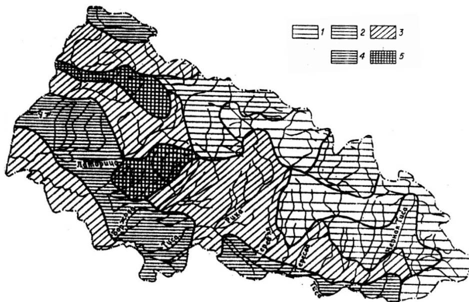
Рис. 4. Розподіл гідроморфологічного коефіцієнту на території Закарпатської області.
