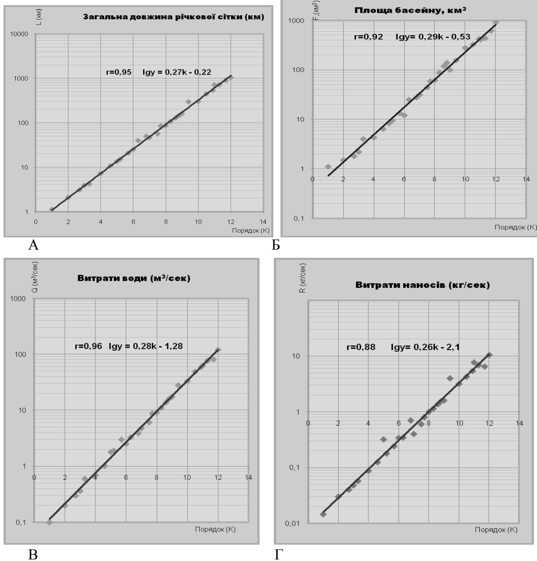
Рис. 3. Зв'язок порядку річкових систем Закарпаття із: А) загальною протяжністю річкової сітки; Б) площею басейнів; В) середньою багаторічно витратою води; Г) середньою багаторічною витратою наносів
