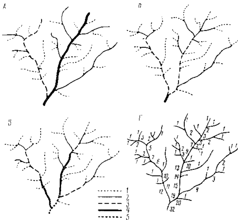
Рис. 1. Класифікація річкових систем за моделями Хортон (А), Штралера (Б), Ржаніцина (В) і Шрива (Г).
